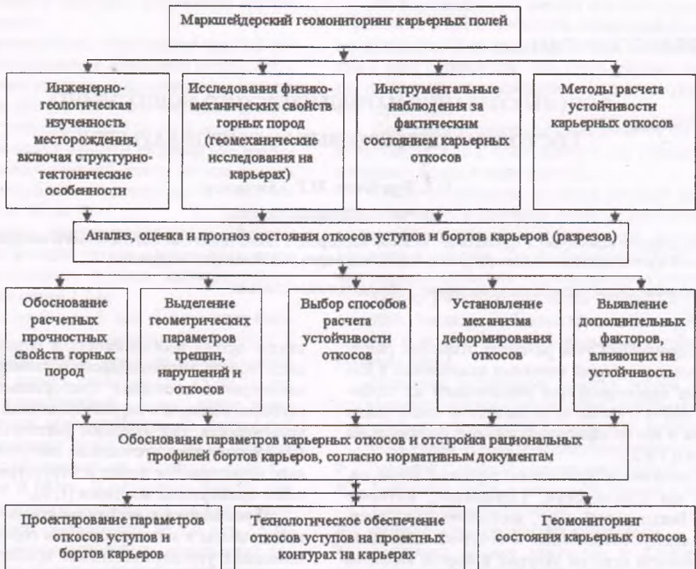
Рисунок 3 – Структурная схема организации геомониторинга прибортовых массивов карьеров
