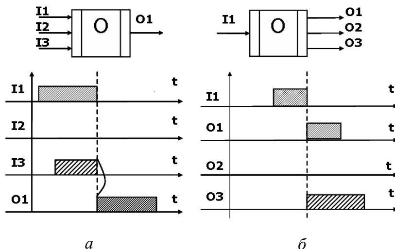
Рис. 2.26. Synchronous OR (Синхронное ИЛИ): а – перекресток слияния; б – перекресток ветвления
