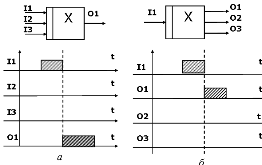
Рис. 2.27. Exclusive OR (исключающее ИЛИ): а – перекресток слияния; б – перекресток ветвления
