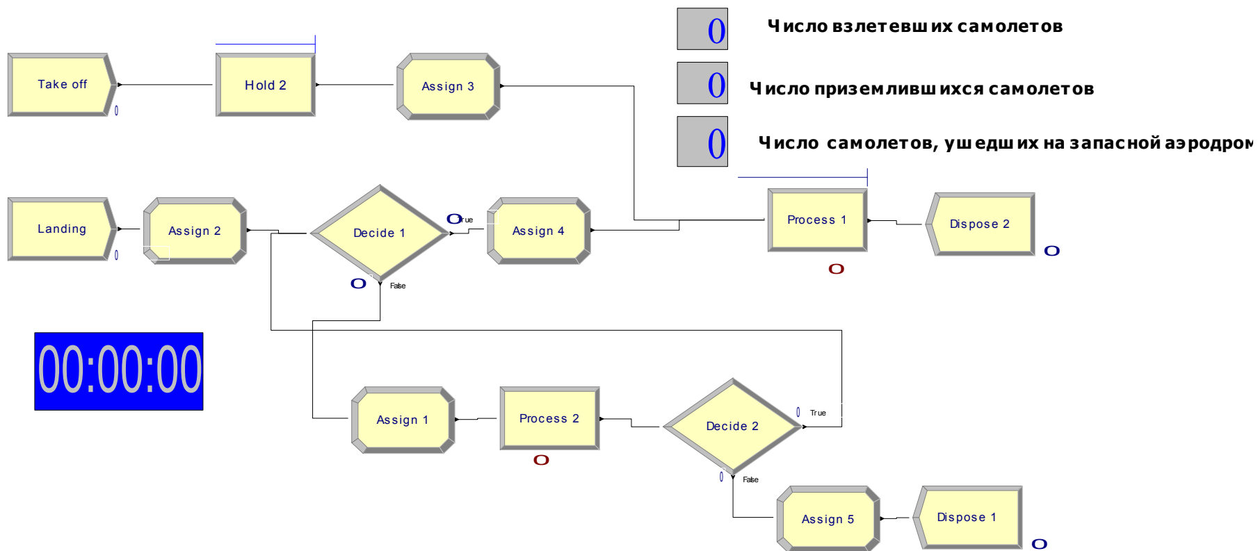
Рис. 3.9. Модель функционирования взлетно-посадочной полосы аэропорта в ПП Arena 7.0
