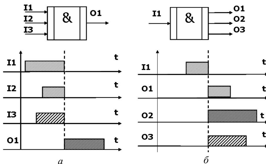
Рис. 2.24. Synchronous AND (Синхронное И): а – перекресток слияния; б – перекресток ветвления
