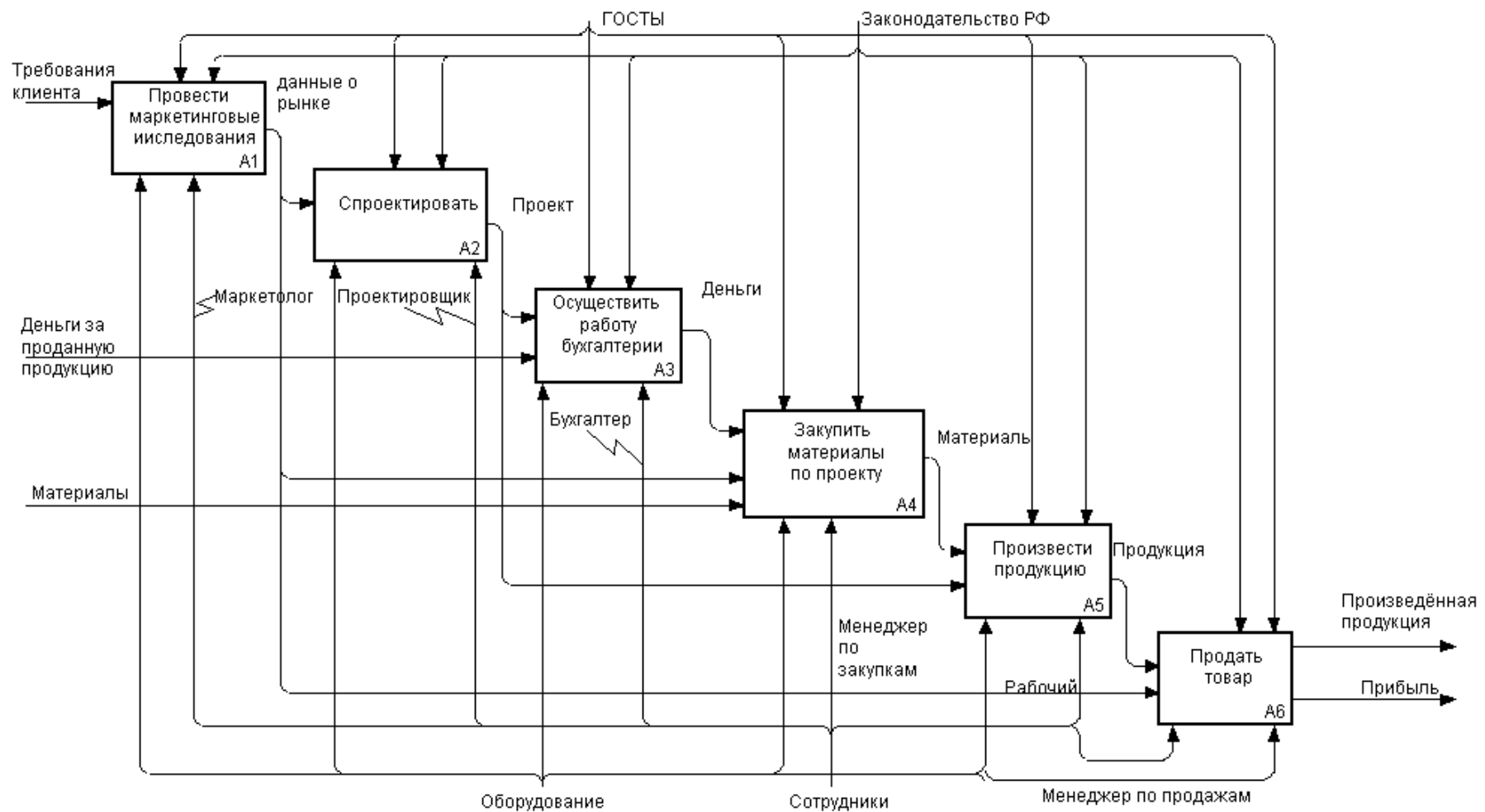
Рис. 2.16. Пример IDEF0-модели деятельности промышленного предприятия:
