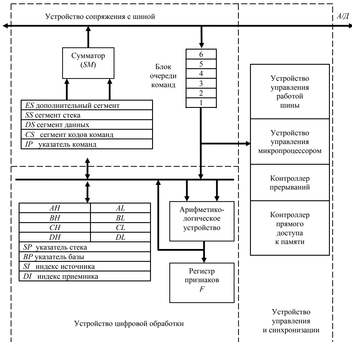
Рис. 2.1 Структура микропроцессора K1810BM86
