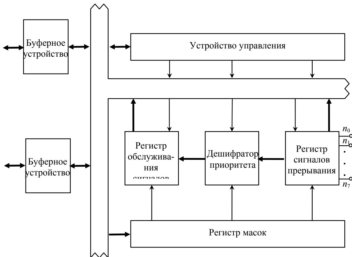
Рис. 1.13 Структурная схема программируемого контроллера прерываний
