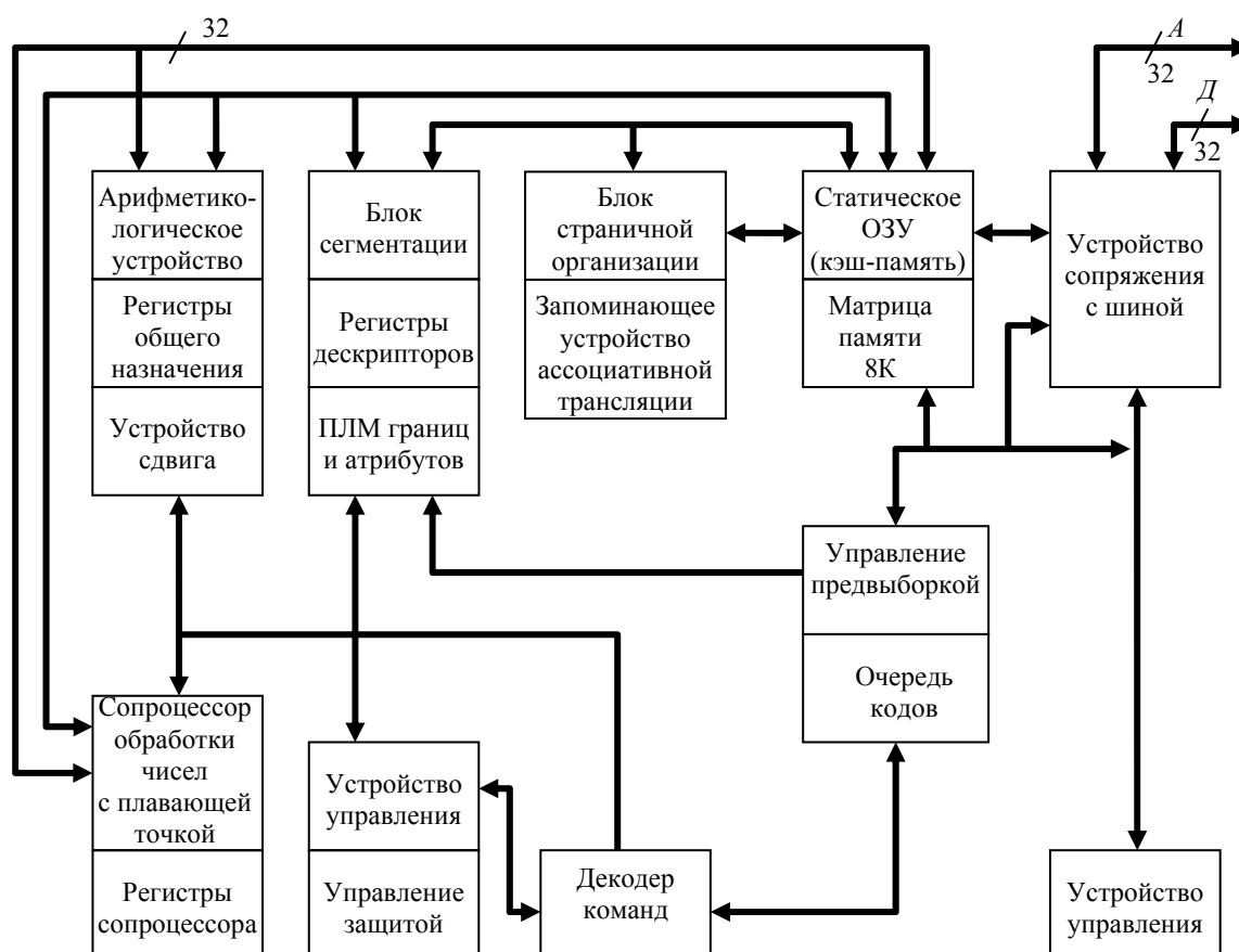
Рис. 2.27 Структурная схема микропроцессора 80486
