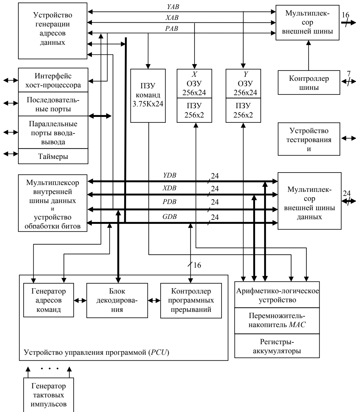
Рис. 3.33 Обобщенная структурная схема цифровых сигнальных процессоров серии DSP56xxx
