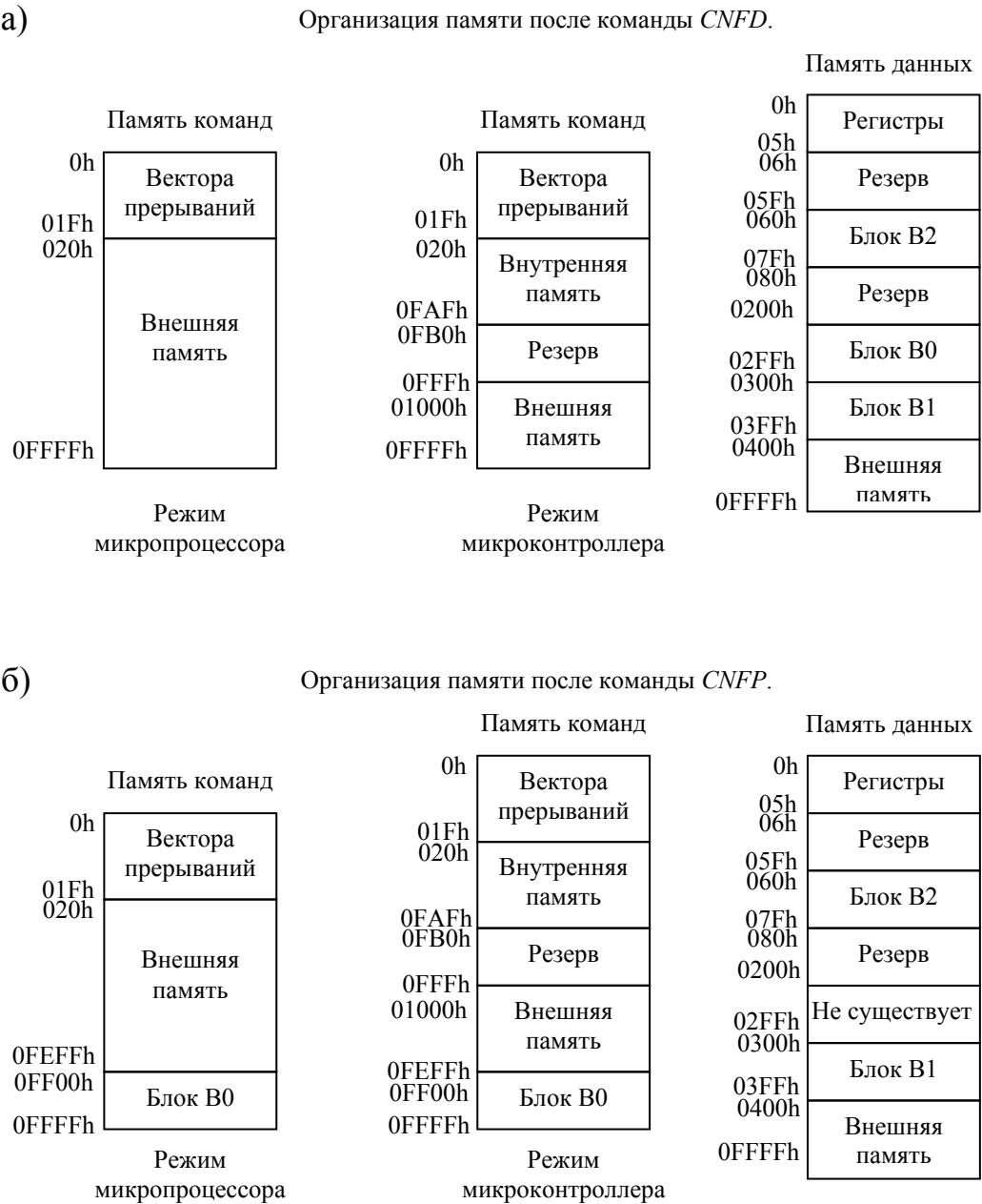
Рис. 9.22 Организация памяти цифровых сигнальных процессоров серии TMS320C2х Использование внутренней памяти команд задается, как и в цифровом сигнальном процессоре TMS320C10 (см.рис.3.20), битом MC/MP , определяющим режим работы как микроконтроллера или микропроцессора. В первом режиме используется внутренняя память, а во втором – применяется
