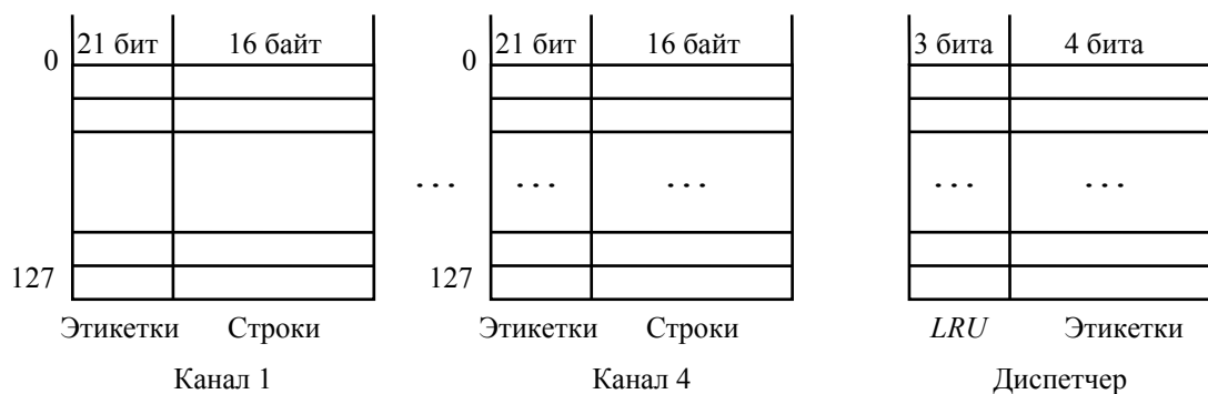
Рис. 2.28 Структура кэш-памяти микропроцессора 80486
