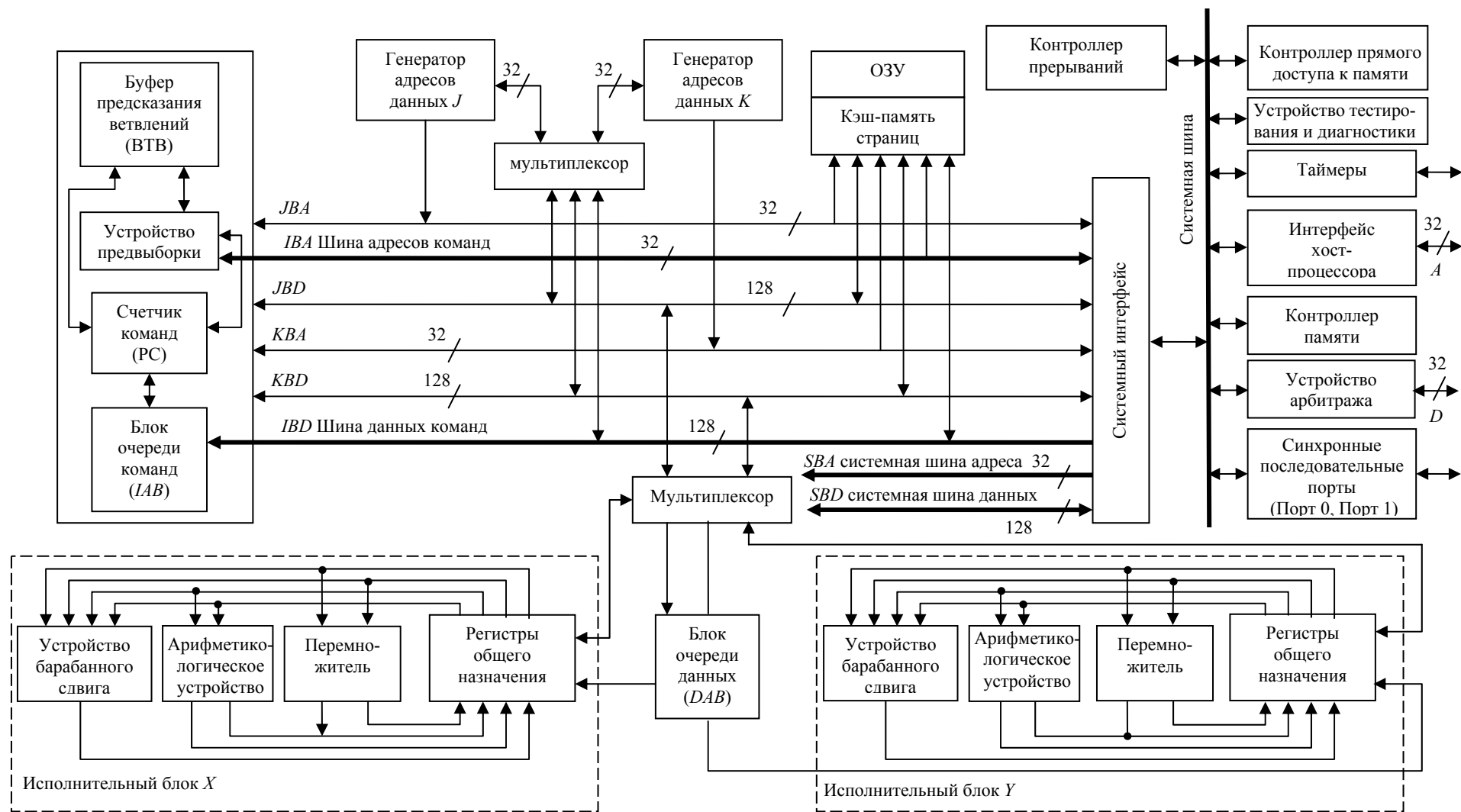
Рис. 3.32 Структурная схема цифрового сигнального процессора ADSP – TS203S
