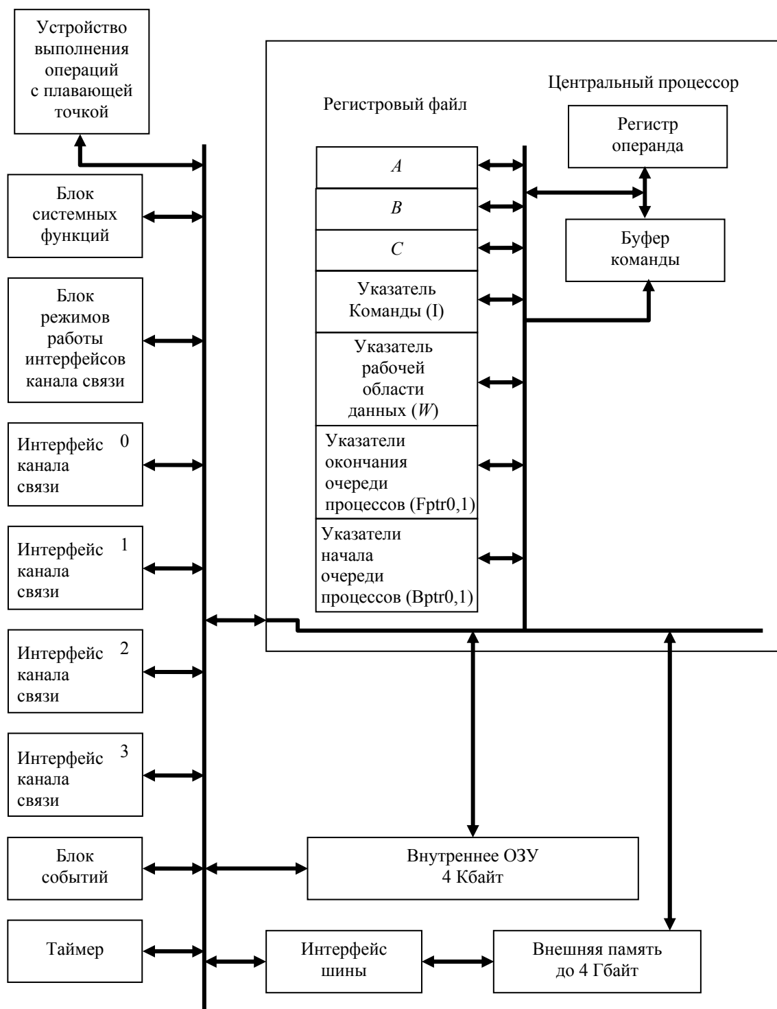
Рис. 2.33. Структурная схема транспьютера T800
