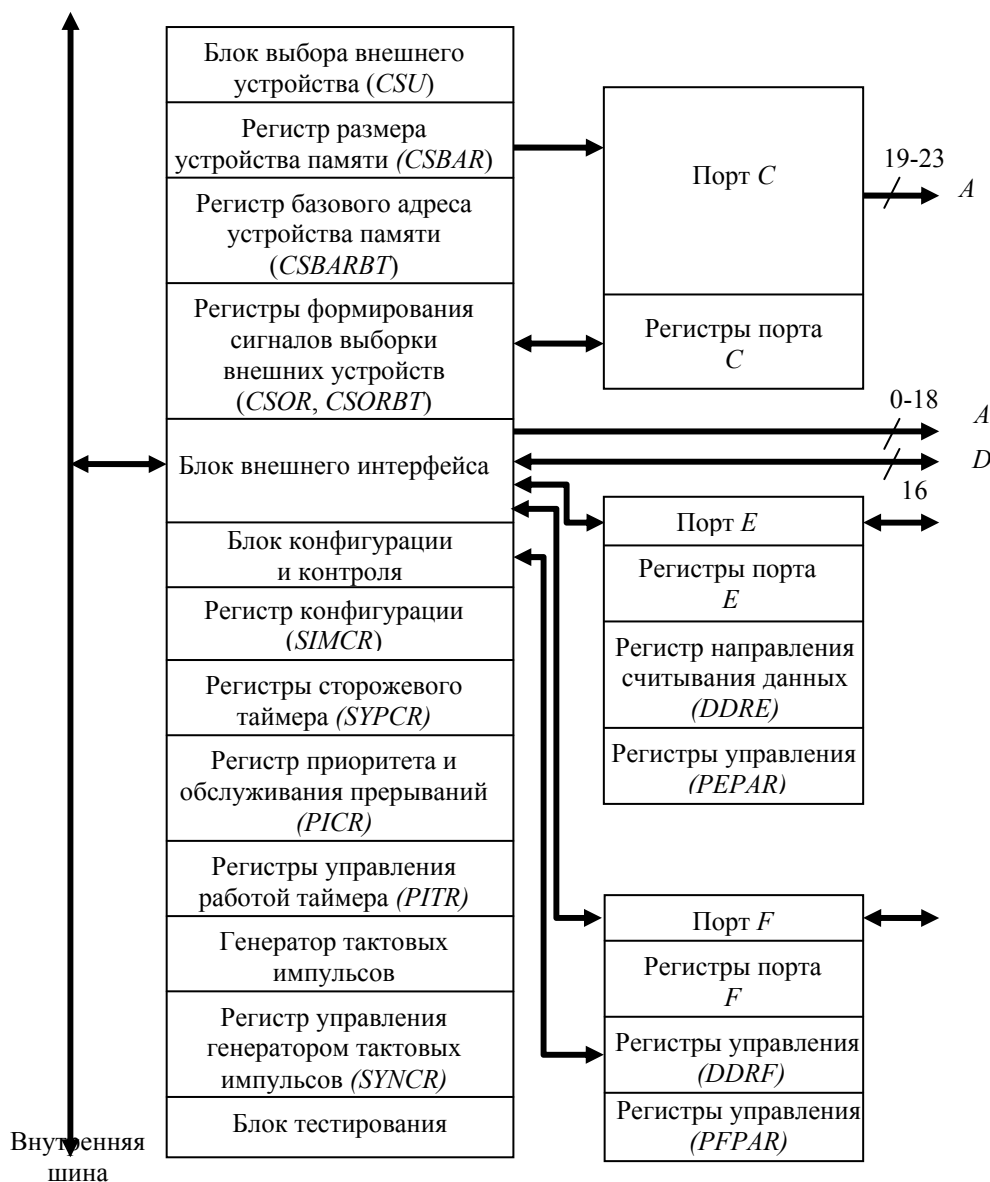
Рис. 3.14 Структура модуля системной интеграции (SIM) 32-разрядного микроконтроллера серии MC683xx
