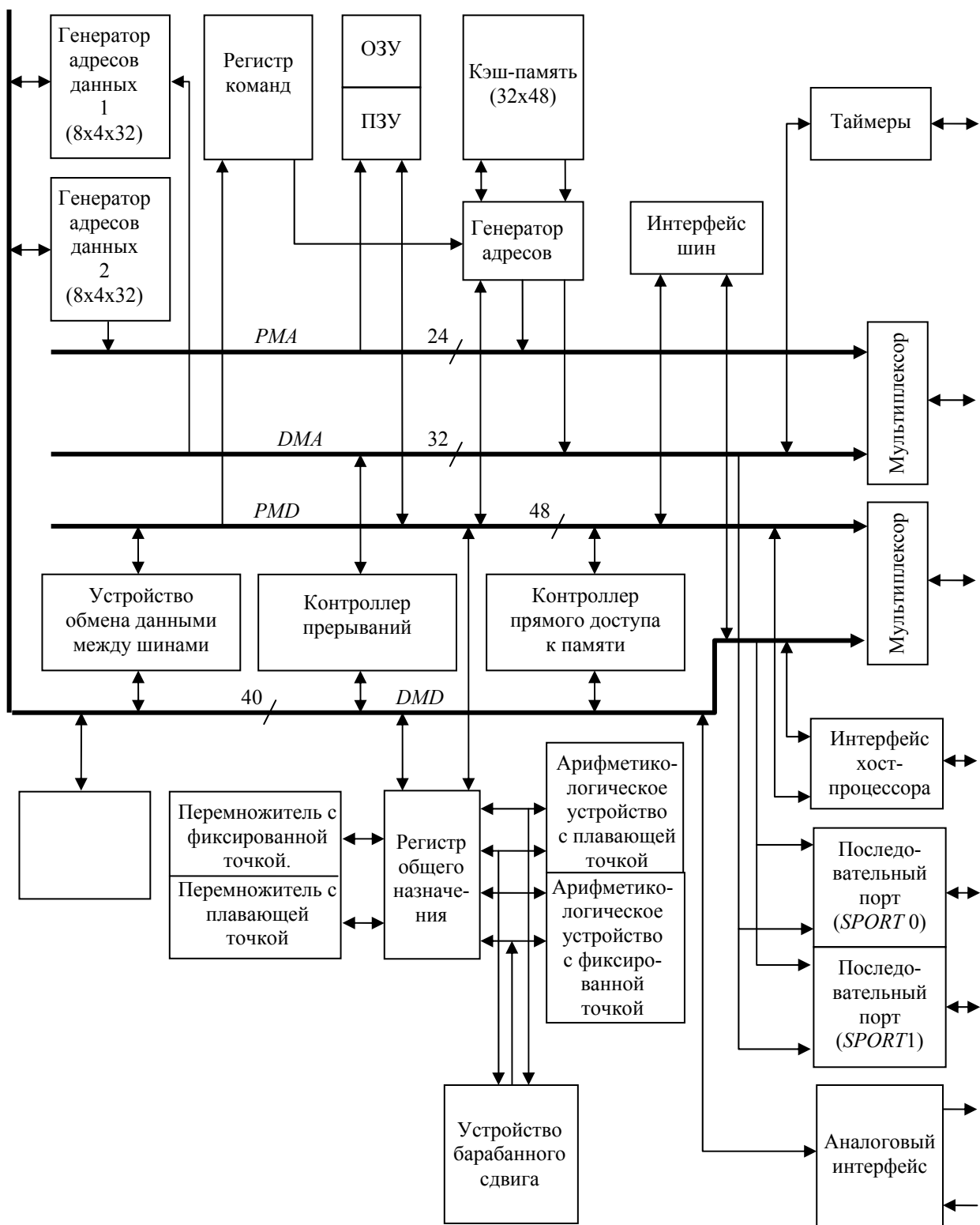
Рис. 3.30 Структура цифрового сигнального процессора ADSP21020
