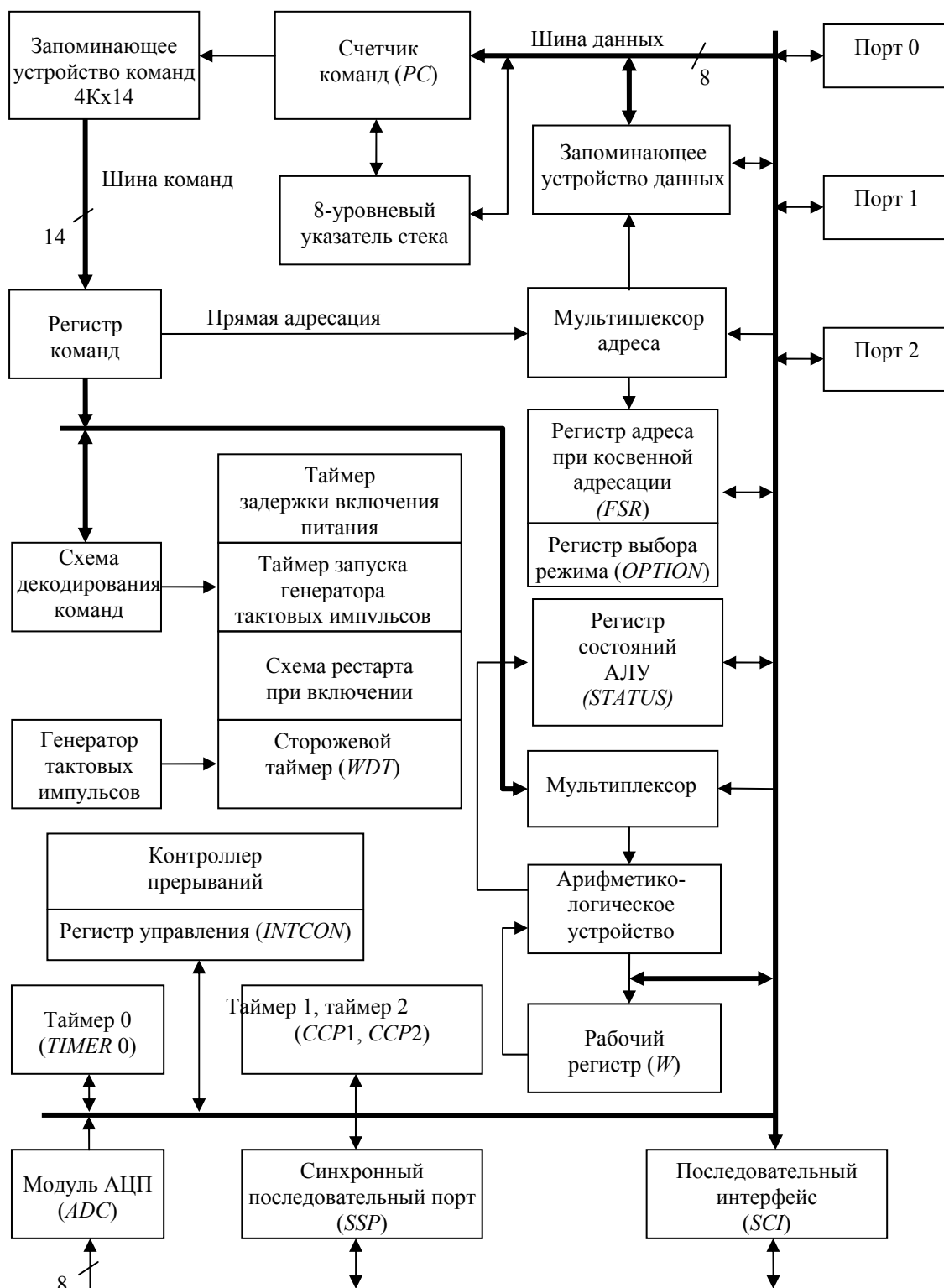
Рис. 3.3 Структурная схема микроконтроллера PIC16C74
