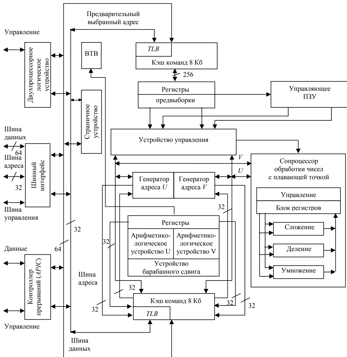
Рис.2.29 Структурная схема микропроцессора PENTIUM
