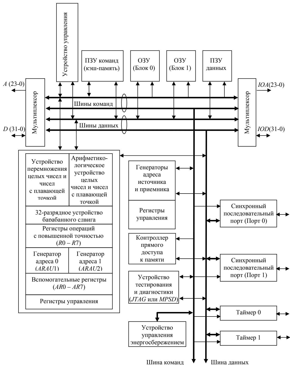
Рис. 3.23 Обобщенная структурная схема цифровых сигнальных процессоров серии TMS320C3x
