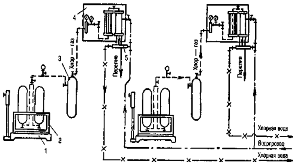
1 – весы; 2 – стойка с баллонами; 3 – грязеуловитель (промежуточный баллон); 4 – хлоратор; 5 – эжектор
