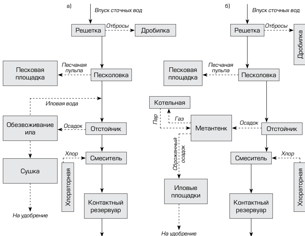
Рисунок 3.2. Схемы станции с механической очисткой сточных вод а – вариант без метантенка; б – вариант с метантенком
