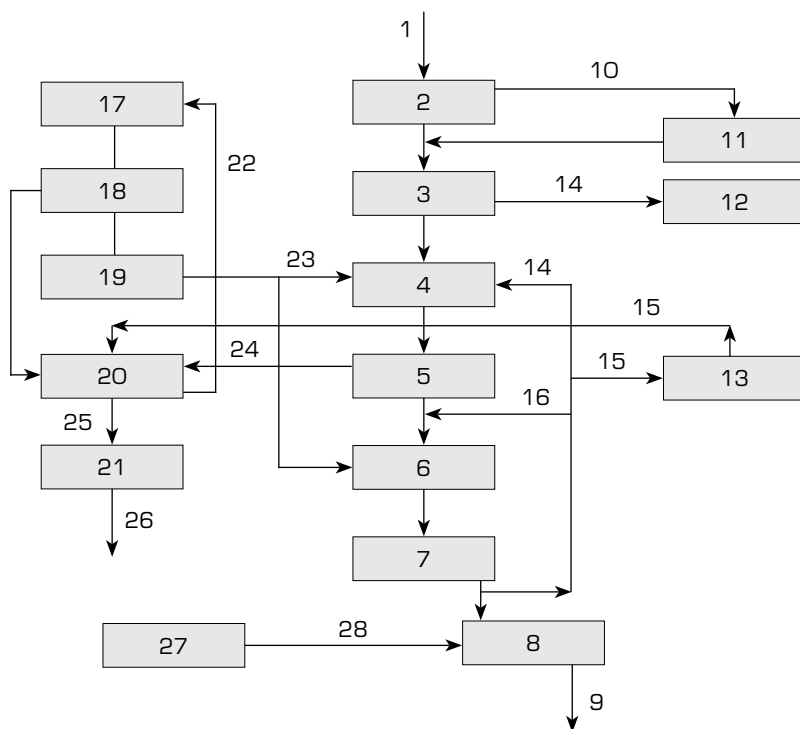
Рисунок 3.3. Схема станции с биологической очисткой сточных вод в аэротенках
