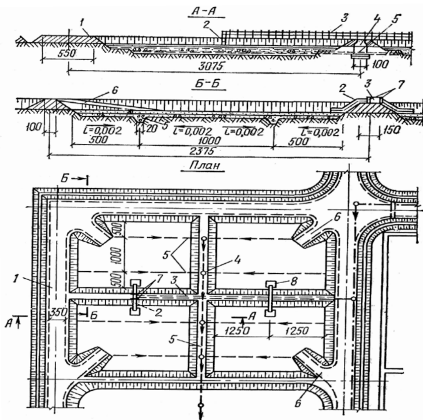
Рисунок 7.3. Иловые площадки
