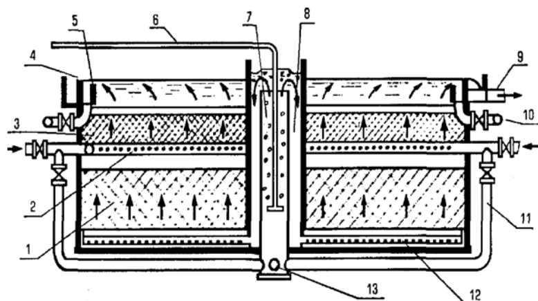
Рисунок 6.3. Биосорбер конструкции ФГУП НИИВодгео
