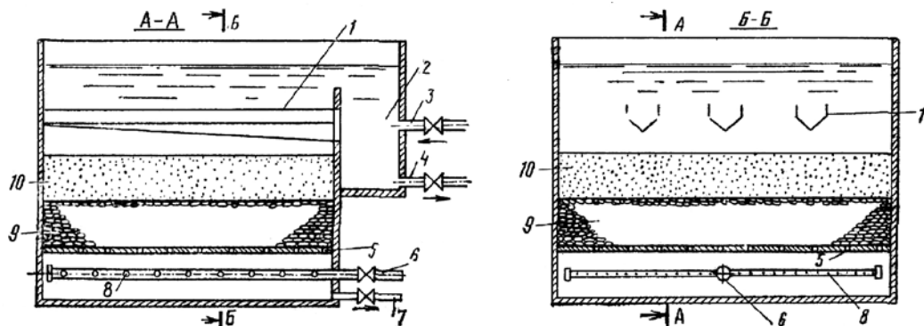
Рисунок 1.5. Однопоточный открытый скорый фильтр
