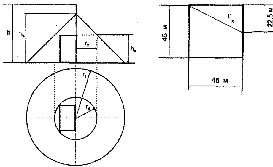
Рисунок 5.3. Схема для расчета молниезащиты
