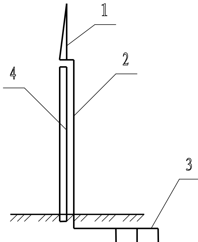
Рисунок 5.1. Устройство молниезащиты
