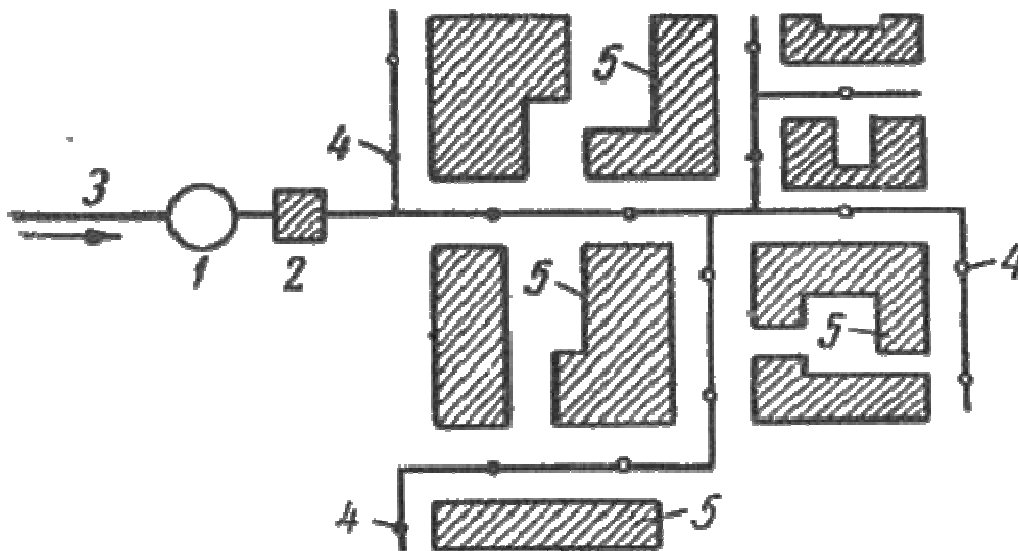
Рисунок 8.2. Схема тупиковой сети водопровода: 1 - запасной резервуар для воды; 2 - насосная станция; 3 - городская магистраль; 4 - гидранты; 5 - здания
