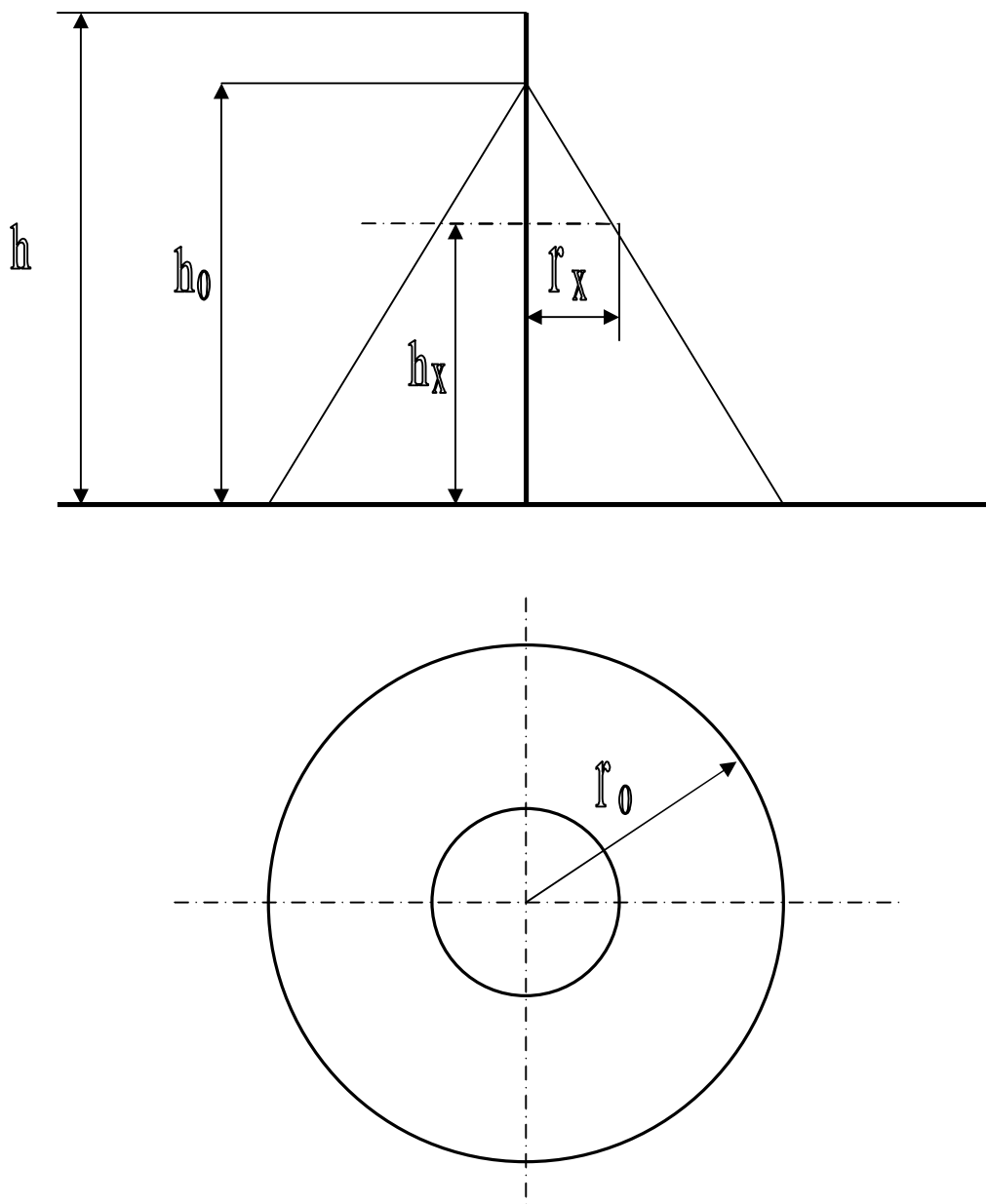
Рисунок 5.2. Зона защиты одиночного стержневого молниеотвода
