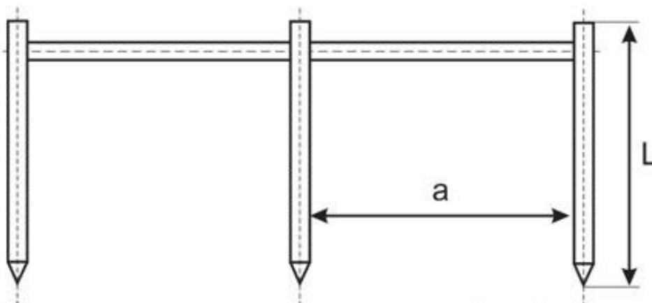
Рисунок 4.3. Схема расположения одиночных стержней заземления
