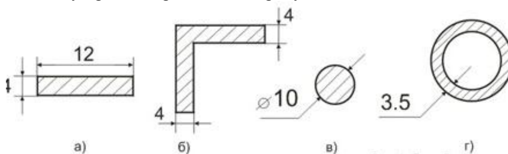
Рисунок 4.1. Минимальные размеры арматуры: а – полоса; б – уголок; в – круглый прокат; в – труба
