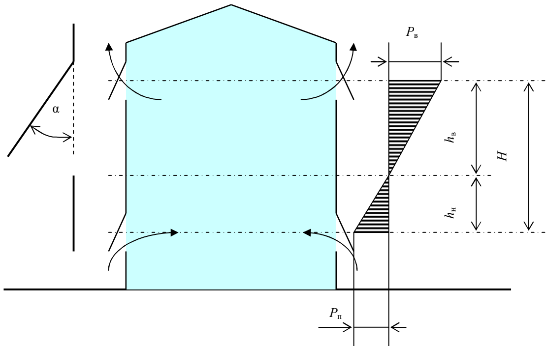
Рисунок 6.1. Схема аэрации производственного помещения
