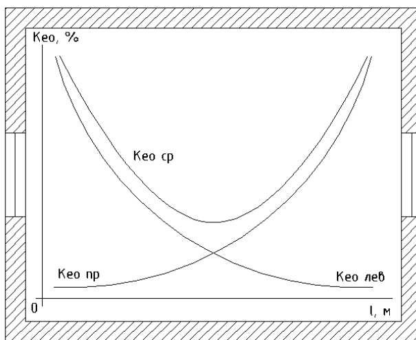
Рисунок 2.2. Боковое двухстороннее естественное освещение
