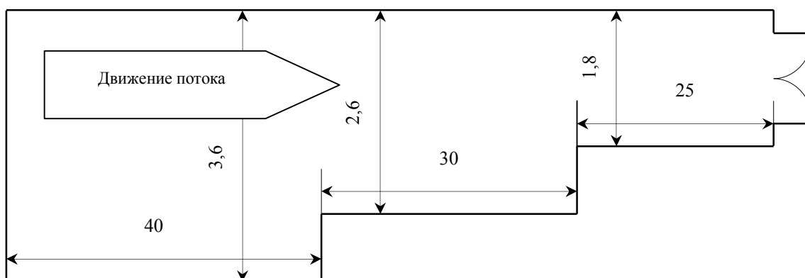
Рисунок 8.3. Расчетная схема эвакуации
