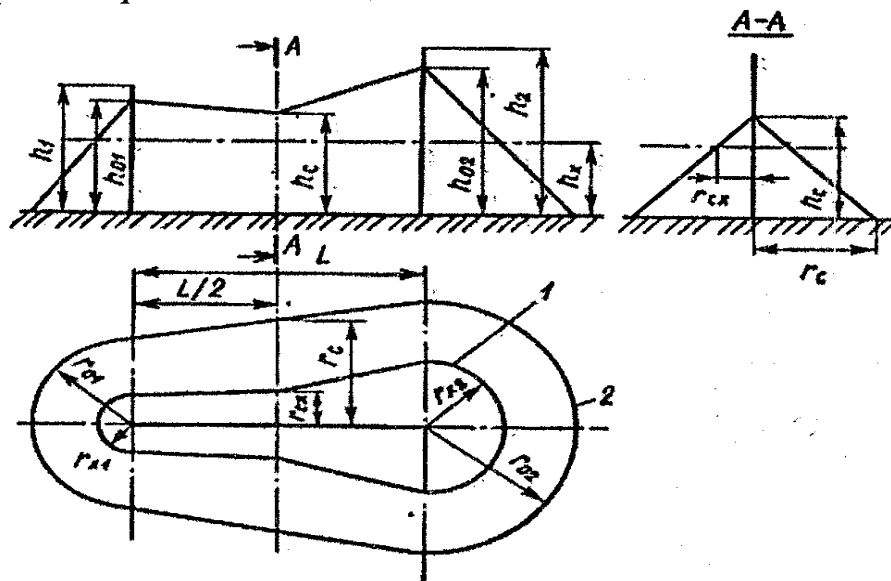
Рис. 5.5. Зона защиты стержневых молниеотводов разной высоты: 1 – граница зоны защиты на уровне h_x ; 2 – то же, но на уровне земли
