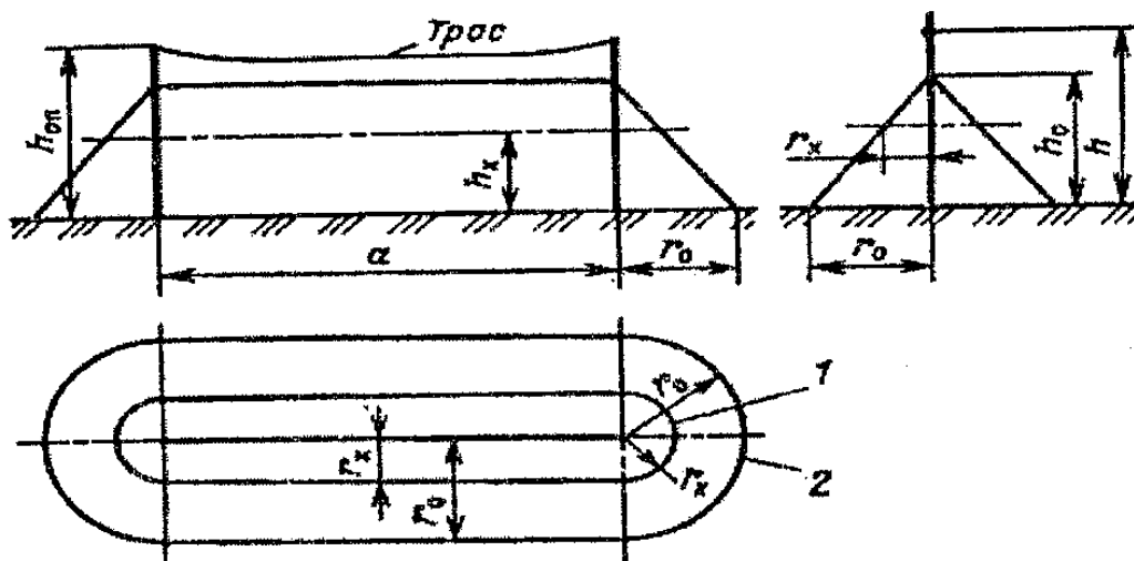
Рис.5.6. Зона защиты одиночного тросового молниеотвода: 1 – граница зоны защиты на высоте h_x ; 2 – то же, но на уровне земли
