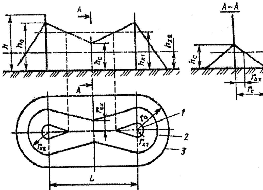
Рисунок 5.4. Зона защиты двойного стержневого молниеотвода: 1 – граница зоны защиты на уровне h_{x1} ; 2 – то же, но на уровне h_{x2} ; 3 – то же, но на уровне земли.
