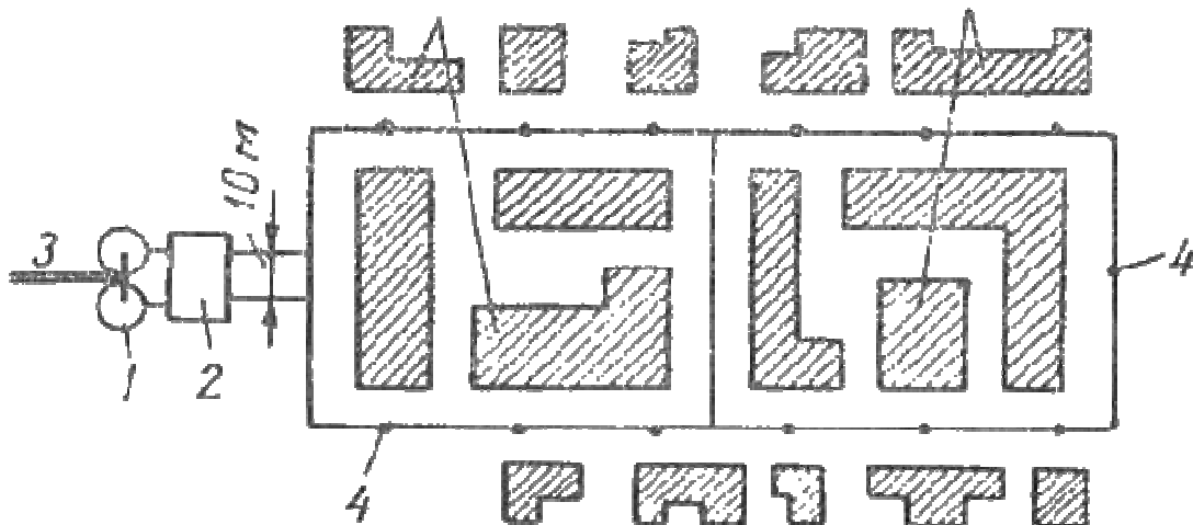
Рисунок 8.1. Схема кольцевого водопровода: 1 - запасные резервуары для воды; 2 - насосная станция; 3 - городская магистраль; 4 - гидранты; 5 - здания
