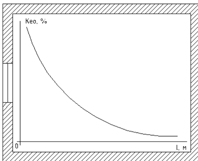
Рисунок 2.1. Боковое одностороннее естественное освещение
