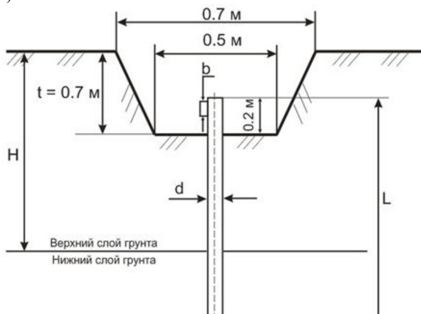
Рисунок 4.2. Схема заложения заземляющего стержня в почву
