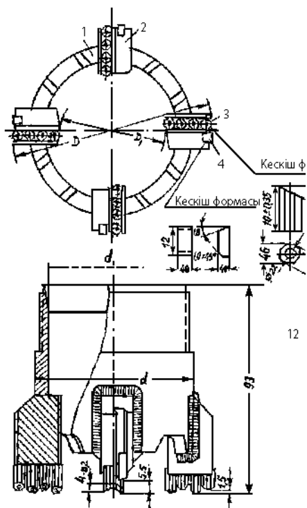
20-сурет. М-5 коронкасы. 1 - тұлға; 2 - кескіштұтқыш; 3, 4 - кескіштер
