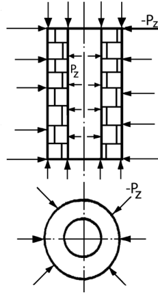
10-сурет. Қуыс цилиндрлерді сынау схемасы
