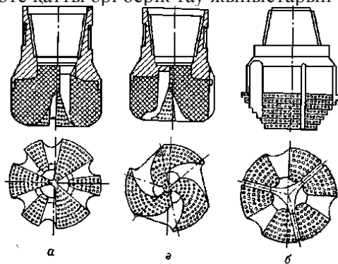
38- сурет. Алмас қашаулар: а – секторлы; в – спиральды; б – сатылы
