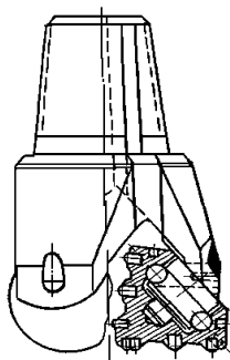
31-сурет. Шарошкалы К типті (бұдыр) қашау
