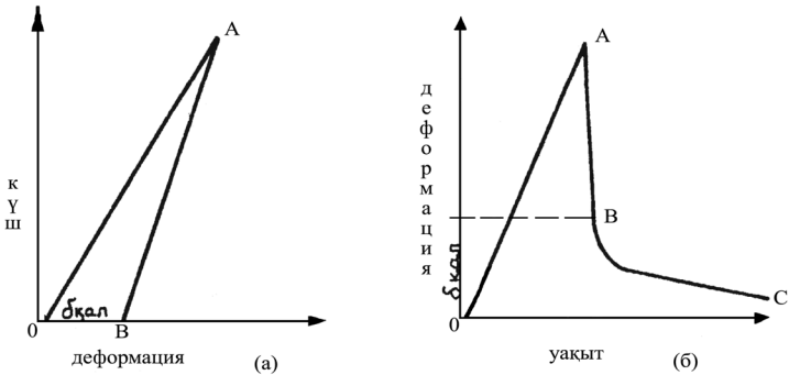
3-сурет. Серпінді гистерезис (а) және серпінділік салдары (б)
