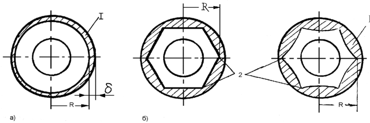
44-сурет. Алмасты коронкалардың корпусы
