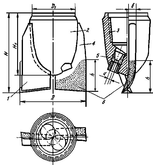
29-сурет. Қос қалақшалы 2Л типті қашау
