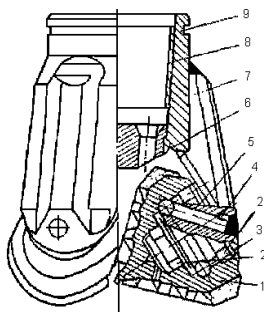
34 - сурет. Тұлғалы қашау: 1 – шарошка; 2 – роликтер; 3 – шар; 4 – штифт; 5 – саусак; 6 – түп темір; 7 – табан; 8 – бұранда; 9 – тұлға
