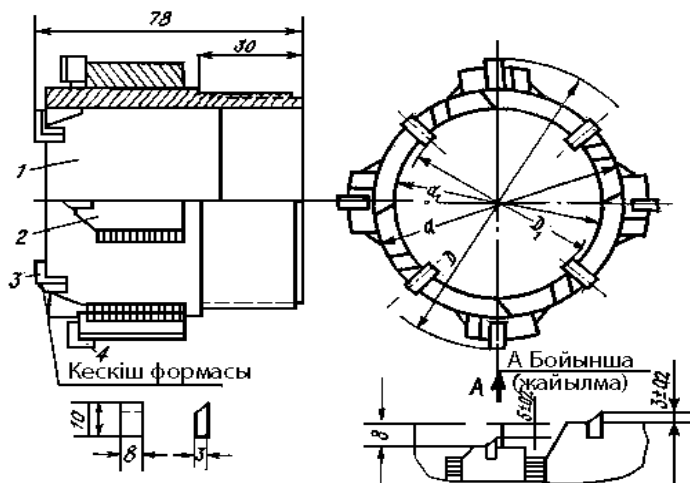
19-сурет. М-1 коронкасы. 1 - тұлға; 2 - кескіштұтқыш қабырға; 3, 4 - кескіштер
