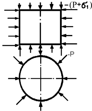
9-сурет. Бокердің схемасымен сынау
