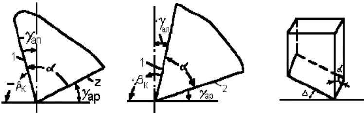
42 – сурет. Кесіп-қопара әсер ететін кескіштердің элементтері
