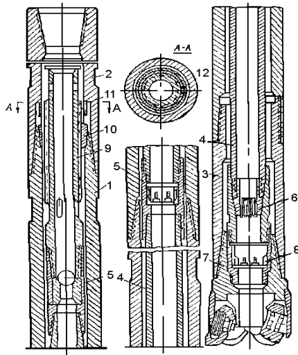
37- сурет. «Недра» колонкалық снаряды
