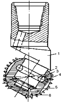
36- сурет. Сыңар шарошкалы қашау: 1 – табан; 2 – шарошка; 3, 5 – шарлар; 4 – саусақ; 6 – қатты қорытпалы кескіштіс
