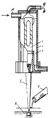
53-сурет. Магнитострикциялық қондырғының схемасы:
