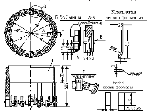
23-сурет. СА-1 коронкасы. 1-тұлға; 2-кемерлегіш кескіш; 3-тіреме пластина; 4-негізгі кескіш; 5-пластина ұстағыш; 6-құйылған жез
