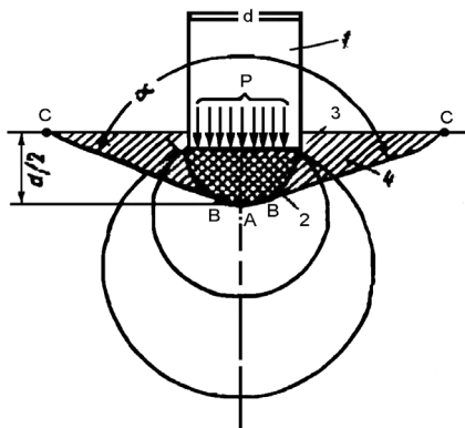
41-сурет. Тау жыныстарын жазық түпті индентормен талқандаудың схемасы
