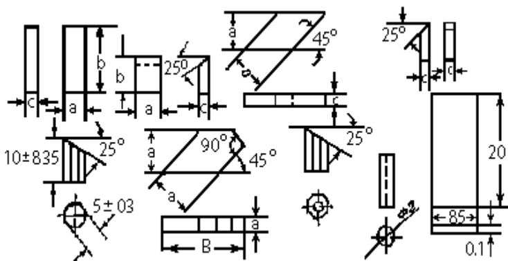
17- сурет. Қатты қорытпадан жасалған кескіштер
