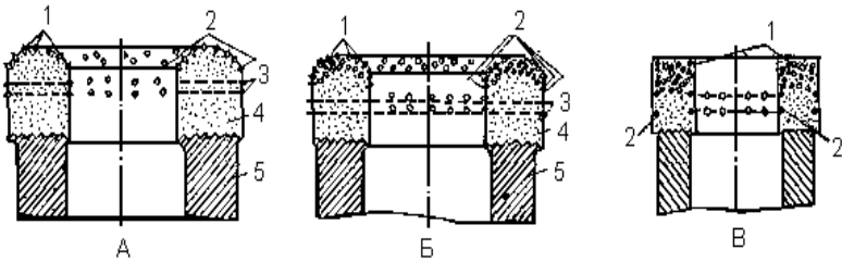
26-сурет. Алмас коронка
