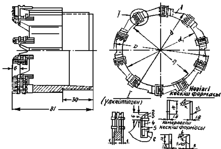
24 – сурет. СА-2 коронкасы. 1 – тұлға; 2 – негізгі кескіш; 3 – кемерлегіш кескіш; 4 – кескіш- тұтқыш; 5 – тіреме пластина; 6 – қондырма пластина
