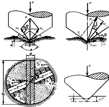
47-сурет. Тау жынысын соққылап талқандаудың схемасы
