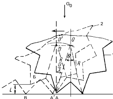
49-сурет. Шарошканың қашаудың жұмыс схемасы:
