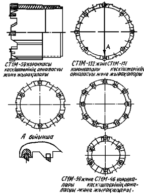
22-сурет. СТ-1М коронкасы
