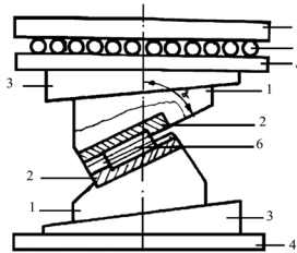
6-сурет. Тау жыныстарының қиюға беріктігін жылжытып сынау арқылы анықтаудың схемасы: 1 – матрица; 2 – қаптама; 3 – сына; 4 – плита; 5 – роликтер; 6 – жыныс үлгісі
