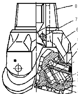
33- сурет. Тұлғасыз қашау: 1 – шарошка; 2 – роликтер; 3 – шар; 4,7 – штифтер; 5 – саусак; 6 – табан; 8 – бұранда
