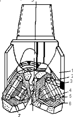
35- сурет. Қос шарошкалы қашау: 1– табан; 2 – саусақ; 3 – штифт; 4 – ролик; 5 – шар; 6 – бірінші шарошка; 7 – екінші шарошка
