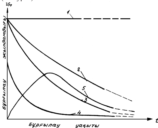
13 сурет. Бұрғылау жылдамдығының бұрғы құралының жұмыс істеу уақытына байланысты өзгеруі. 1 - өздігінен қайралатын құрал; 2,3,4 - қажалып мұқалған құралдар; 5 - геометриялық формасы мен өлшемін өзгертетін құрал (шойын бытыра)
