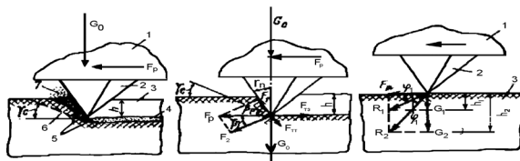
46- сурет Үшкір алмас кескіштің жұмыс схемасы:
