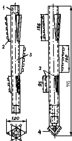
28- сурет. В. П. Новиковтың найза бұрғысы
