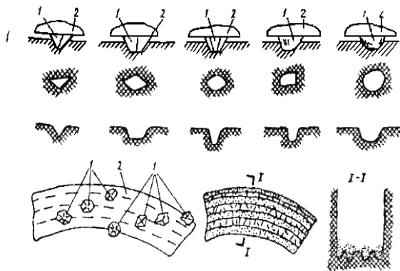
45-сурет. Алмас кескіштердің және тау жынысының талқандалуы нәтижесінде пайда болған ойшықтардың кескіні: 1 - алмас түйіршіктері; 2 - коронканың матрицасы
