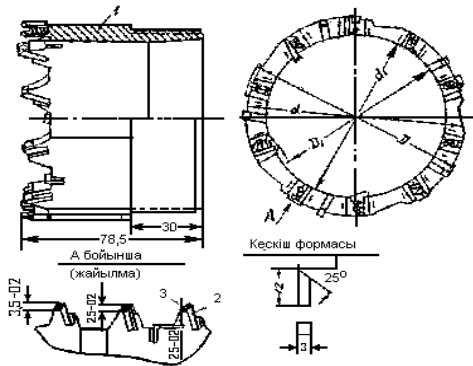
25-сурет. СА-4 коронкасы. 1 – тұлға; 2 – кескіш; 3 – құйылған жез
