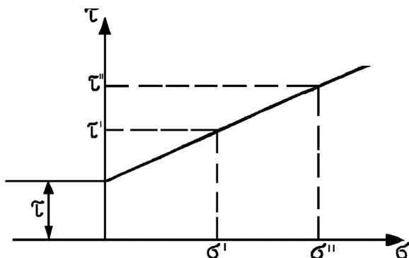
7-сурет. \sigma = 0 сәйкес болғандағы қиюға қарсылықты анықтау графигі
