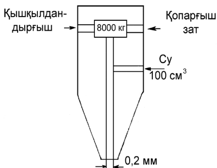
54-сурет. Островскийдің құралы
