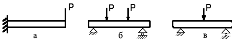
5-сурет. Үлгілерді майыстырып сынау схемалары
