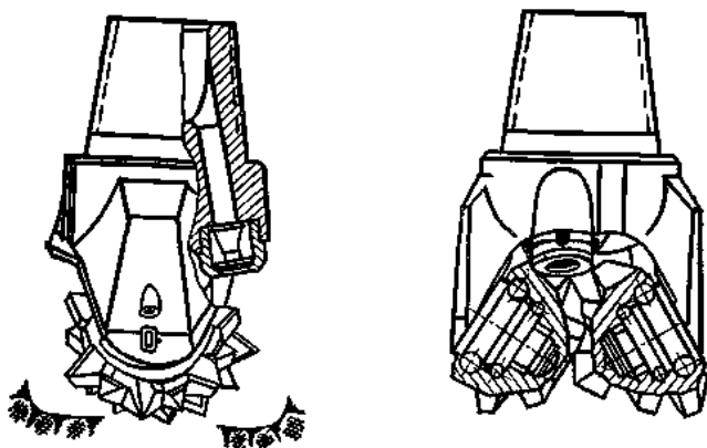
30-сурет. М типті шарошкалы қашау
