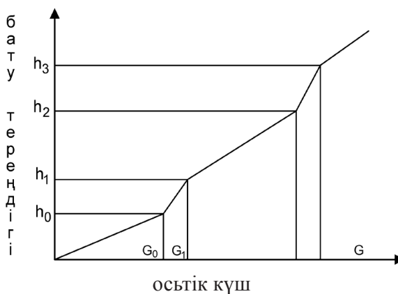
51-сурет. Айналсоқ әдісте осьтік күш пен индентордың бату тереңдігінің арасындағы байланыс
