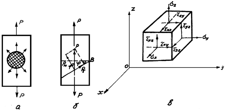
1- сурет. Үлгіде кернелген жағдай туғызатын күштердің әсер ету схемасы
