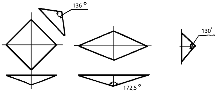
11- сурет. Алмас пирамидалар
