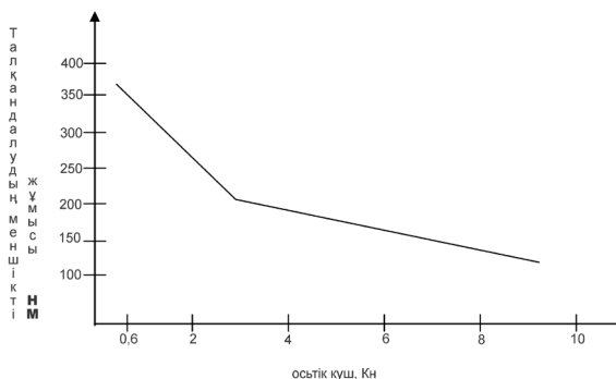
52-сурет. Талқандаудың энергия сыйымдылығының осытік күшке байланысты өзгеруі
