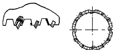
СММ 132 және СММ-151 коронкалары кескіштерінің орналасуы
