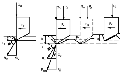
50-сурет. Осытiк кiштiң, динамикалық кiштiң әсерiмен кескiштiң жұмыс iстеу схемасы
