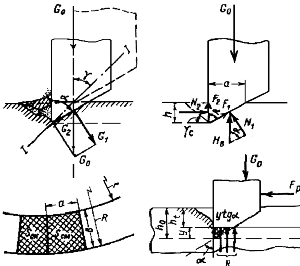
43-сурет. Кескіштің тау жынысына батудағы жұмысының кинематикасы
